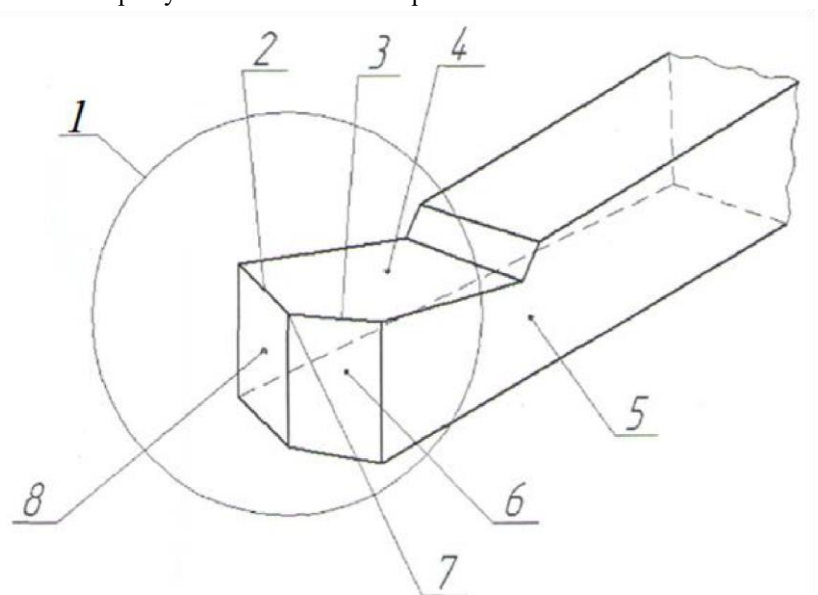
Рис. 4 Элементы резца
